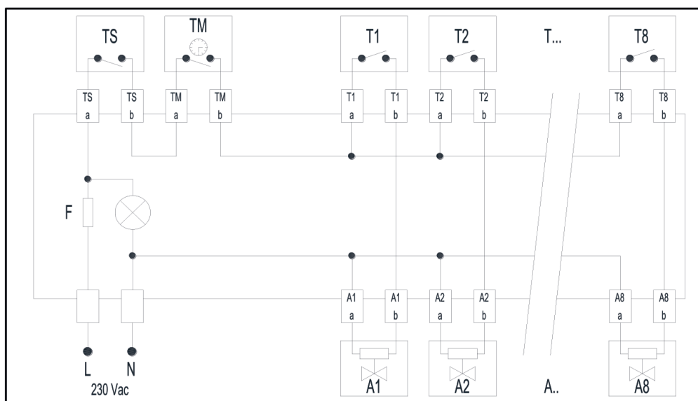
schema collegamenti elettrici
