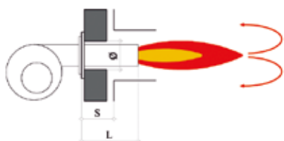
TIPOLOGIA AD INVERSIONE DI FIAMMA
